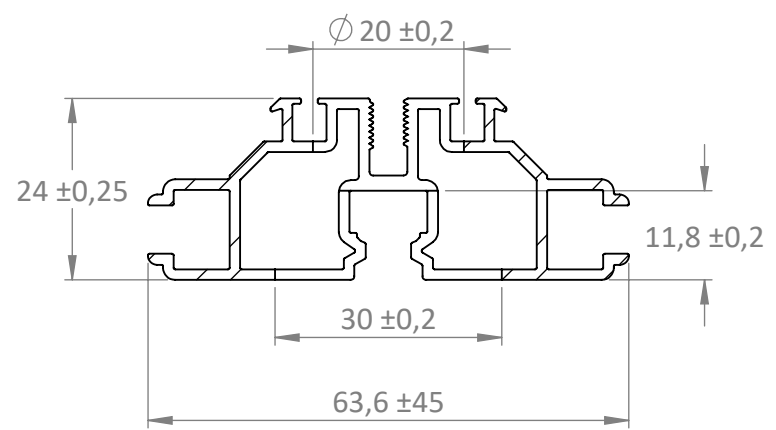
COUPE B-B
