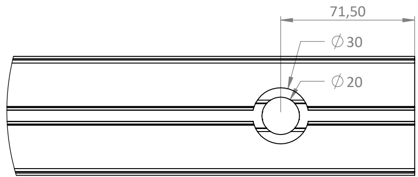
DÉTAIL A
