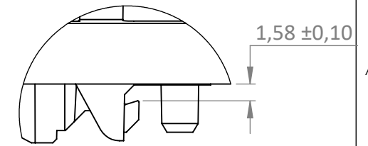
DÉTAIL B ECHELLE 2 : 1
